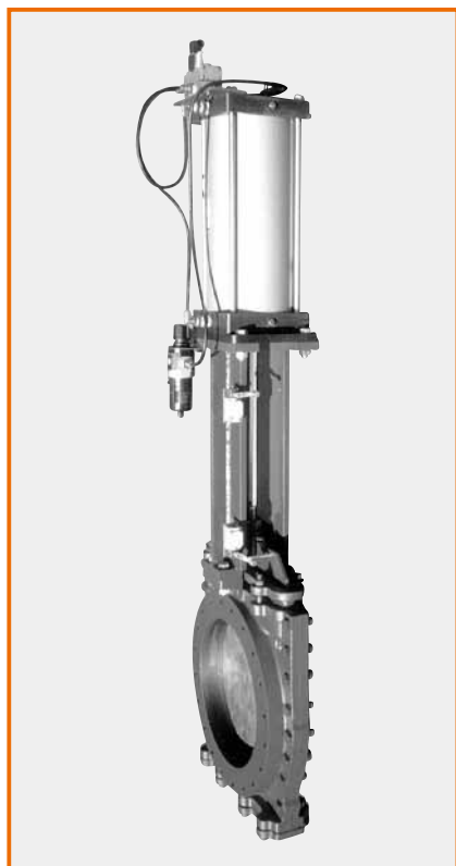
■ショート型板弁 エアシリンダー操作 電磁弁、エア-3点セット付 S-1075
