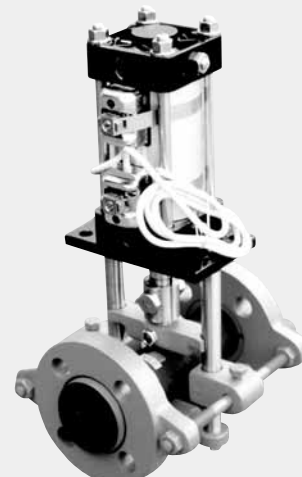
■エアシリンダー操作 S-1531 リミットスイッチ付
