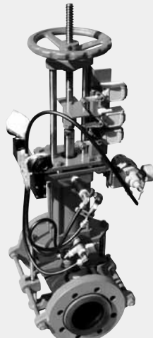
■手動兼エアシリンダー操作 S-1537
