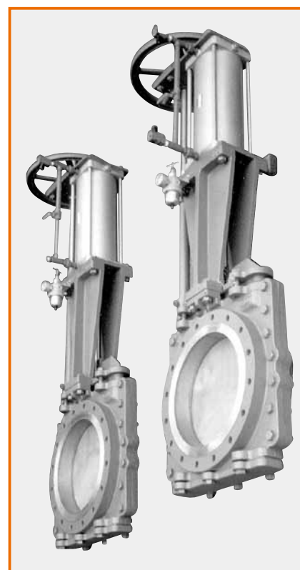
■ショート型板弁 手動兼エアシリンダー操作 スピコン、エアセット付 S-10705
